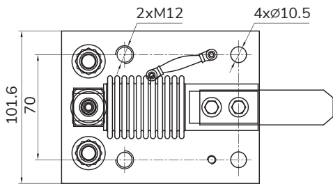
Mounting / 安装示意图
